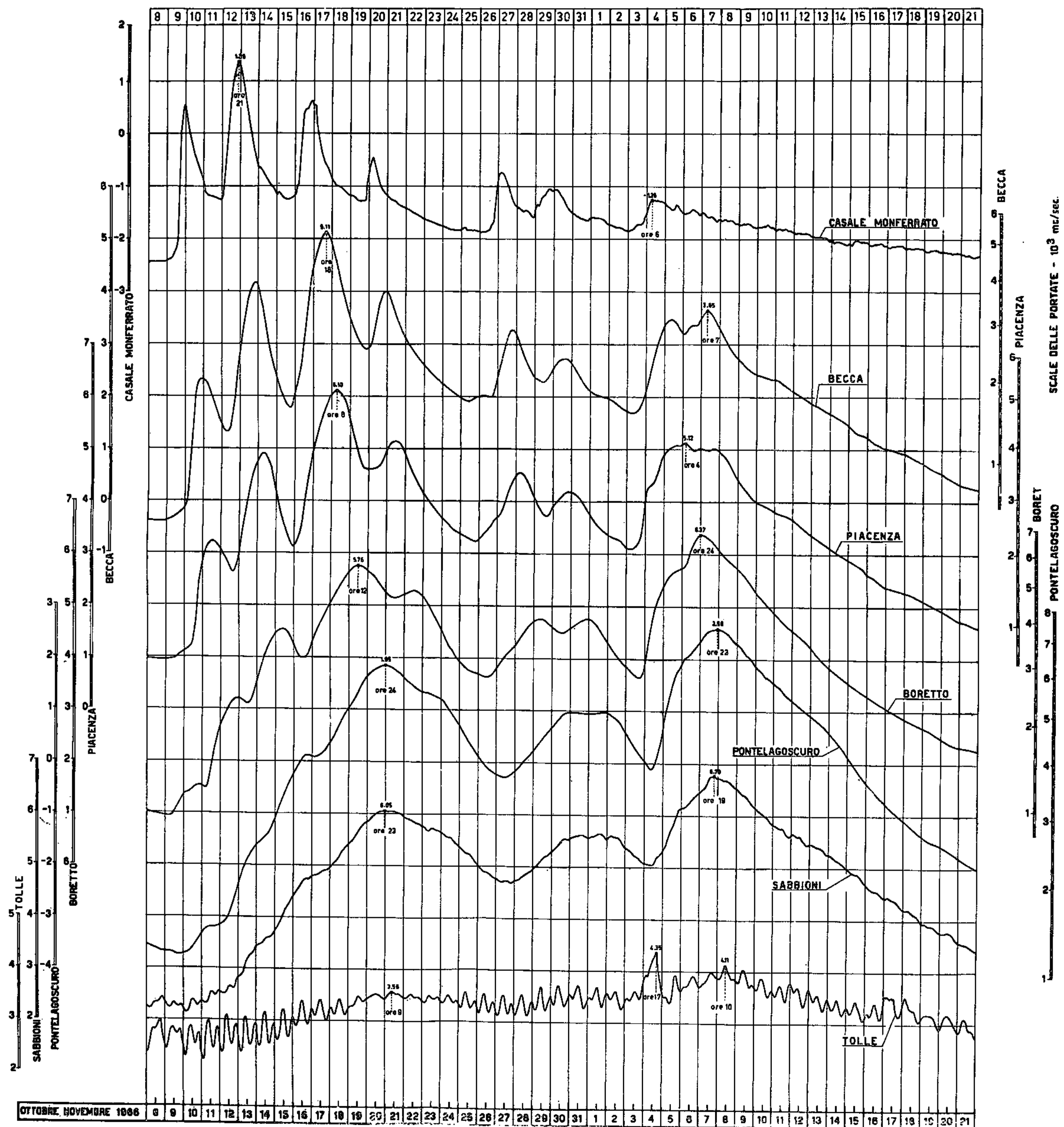
Fig. 14 — F. Po, diagrammi idrometrici dell'ottobre e novembre 1966.
