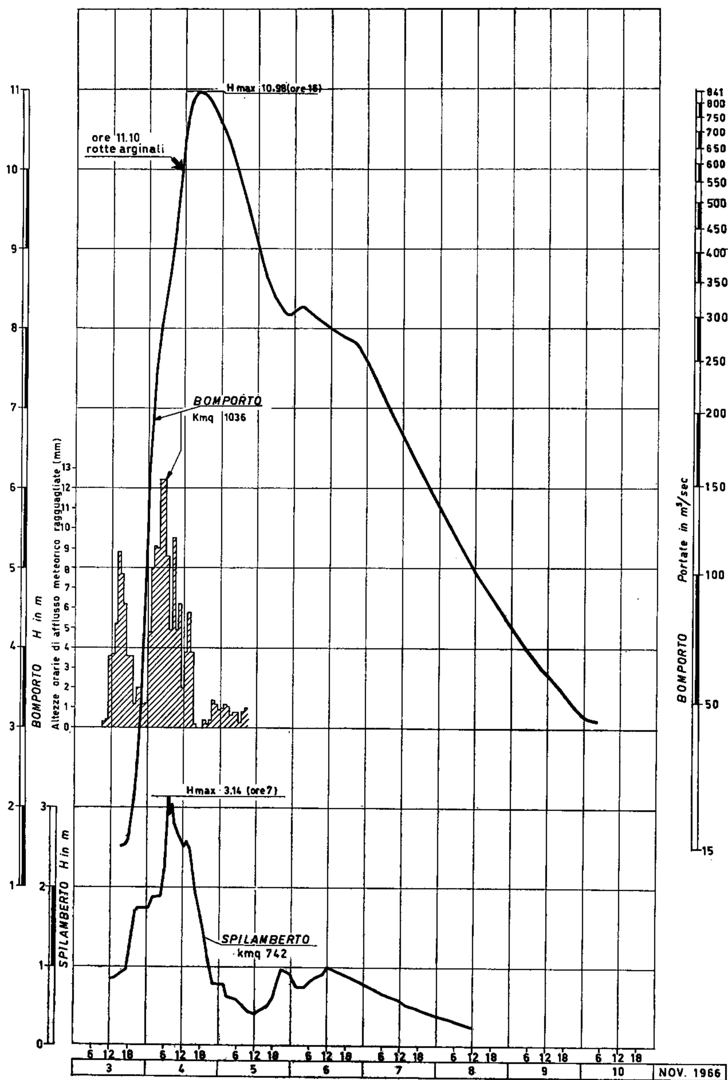
Fig. 13 — Onda di piena del F. Panaro.
