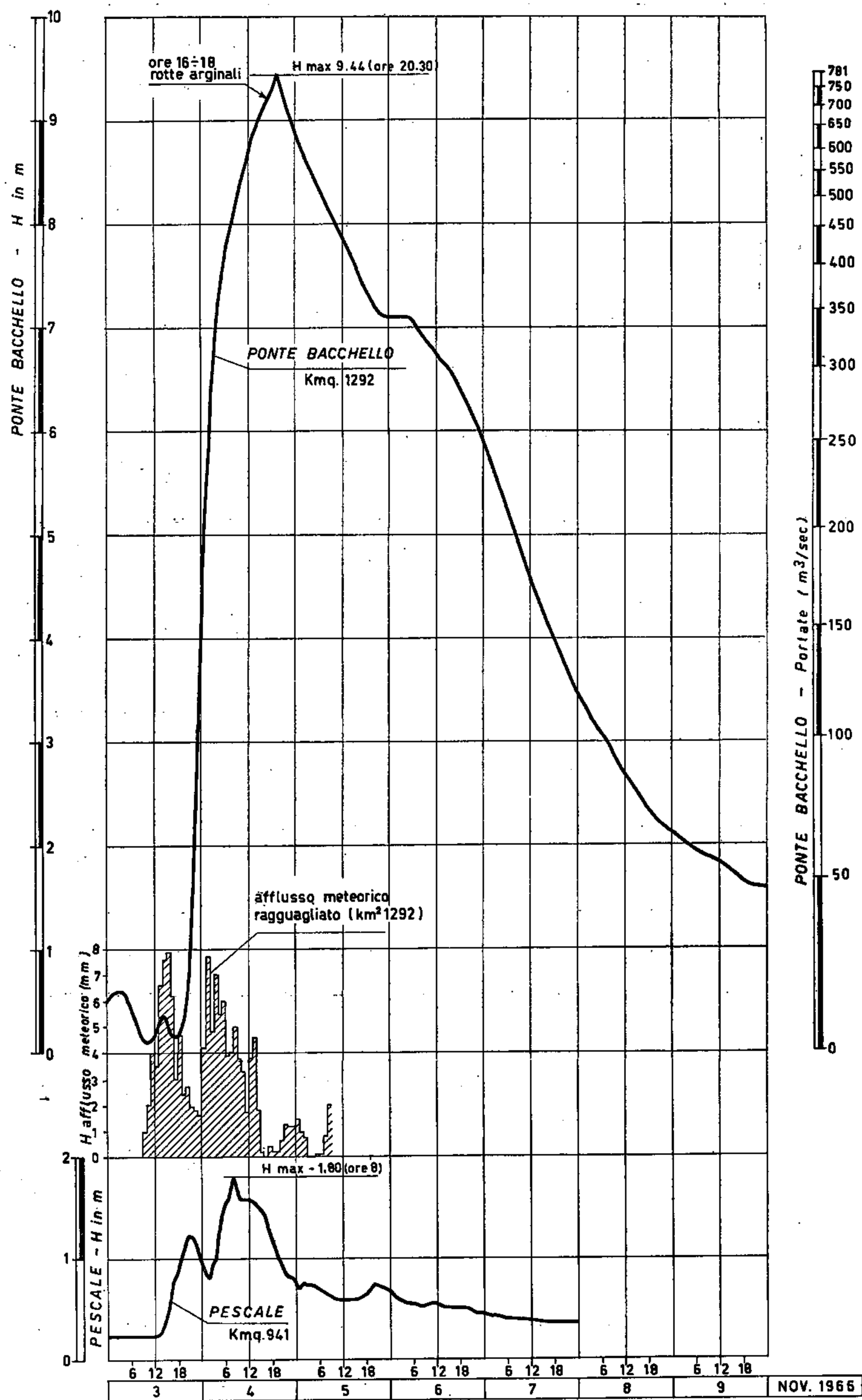
Fig. 12 — Onda di piena del F. Secchia.
