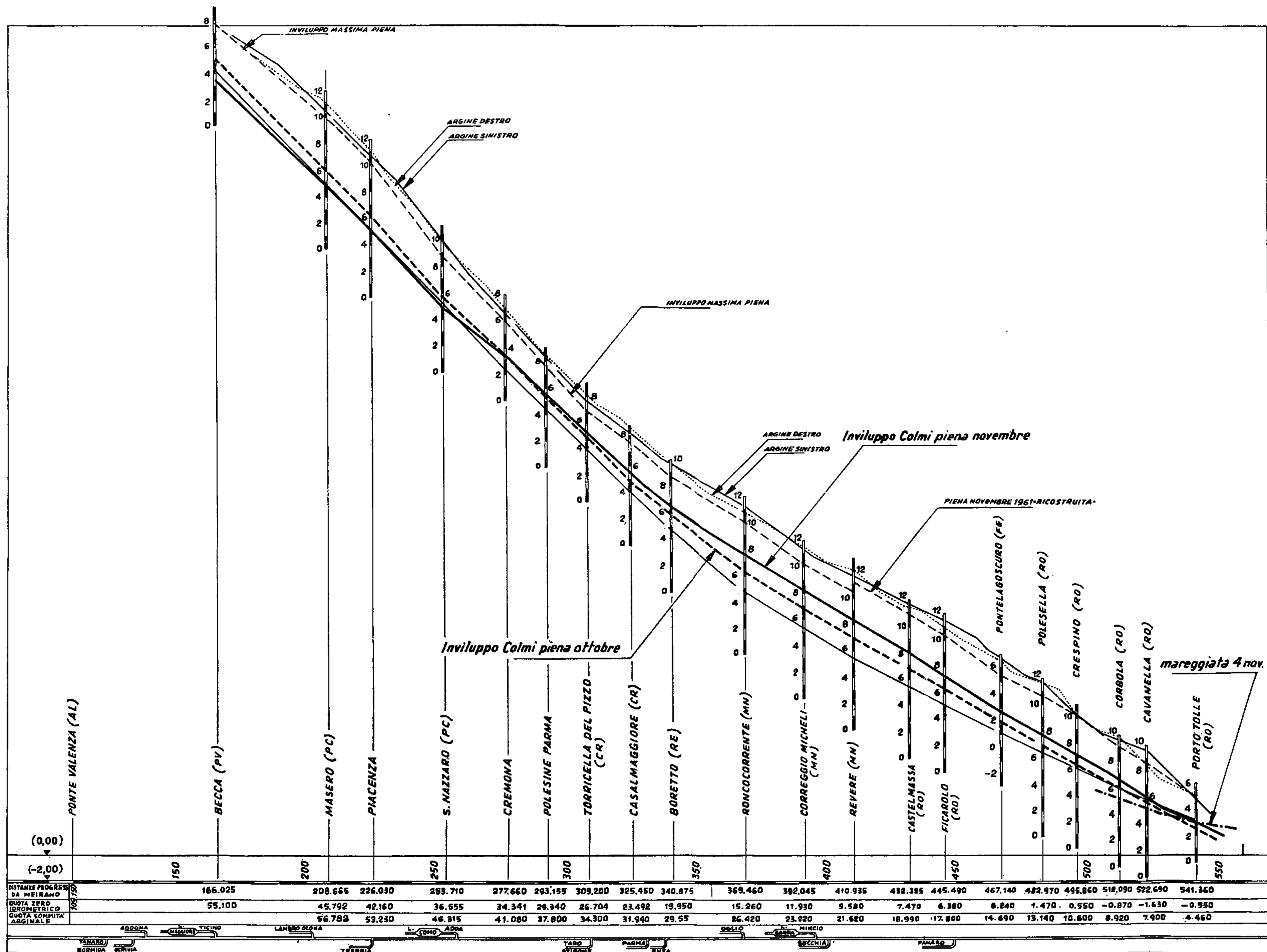
Fig. 15 — F. Po, Profili involucro colmi di piene dell'ottobre e novembre 1966.
