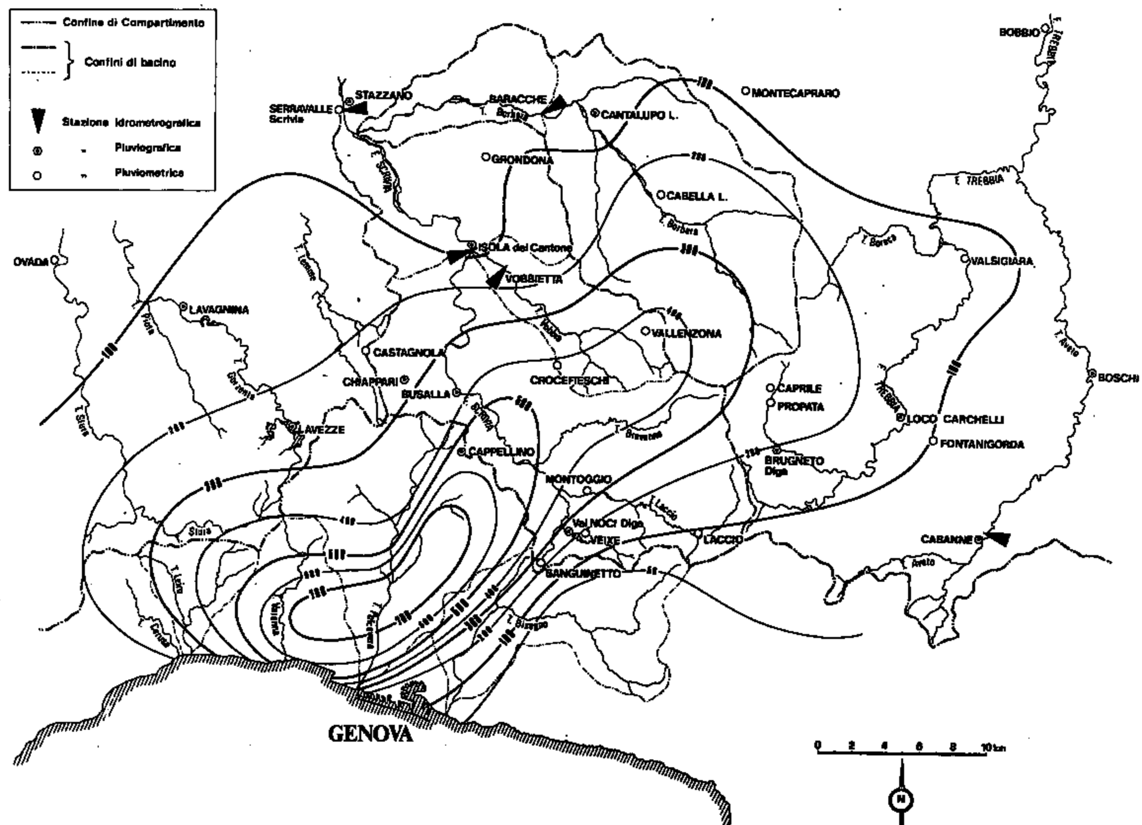
• Carta delle isoiete del giorno 8 ottobre 1970
