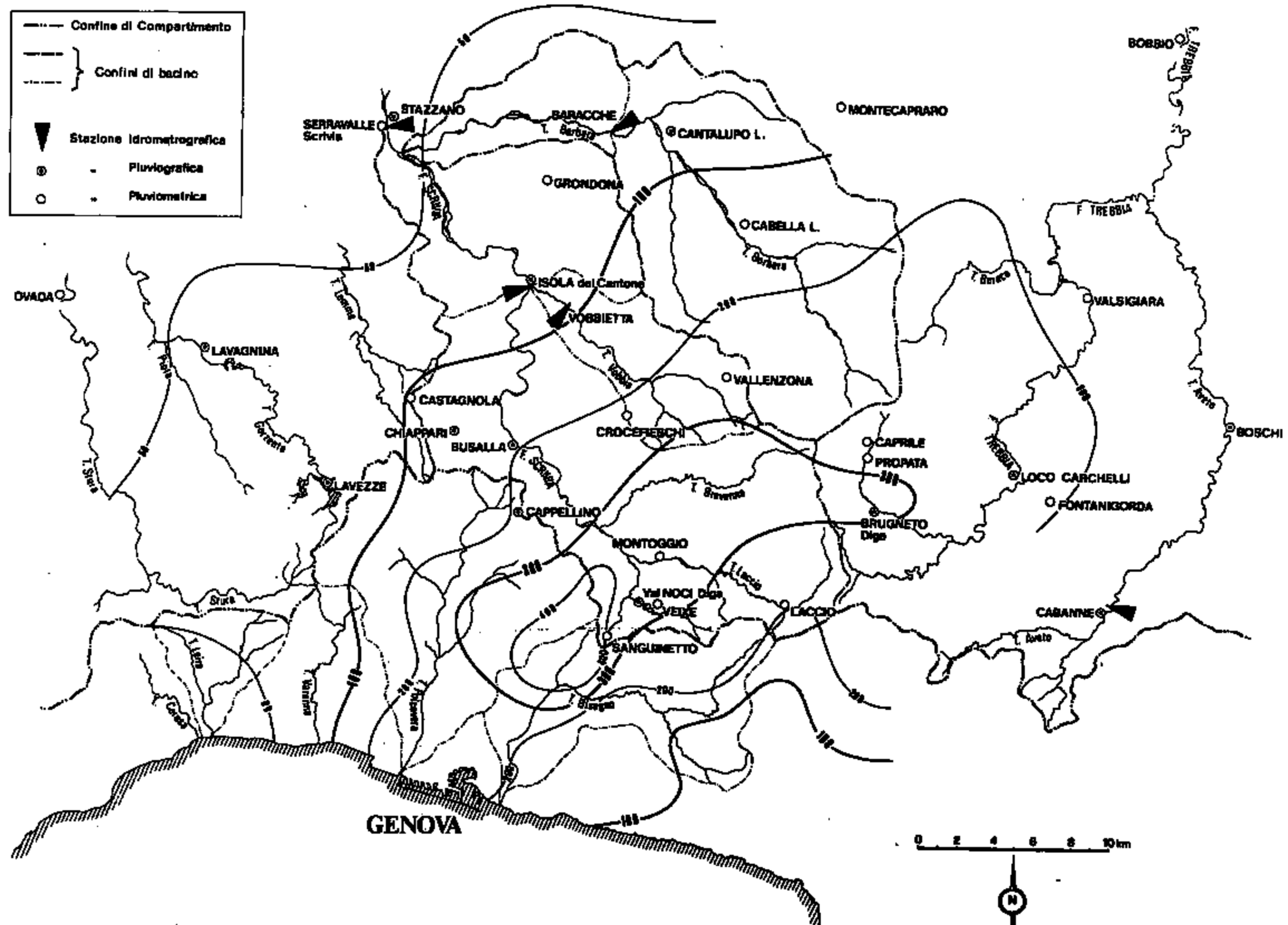
Fig. 2 - Isoiete del giorno 9 ottobre.
