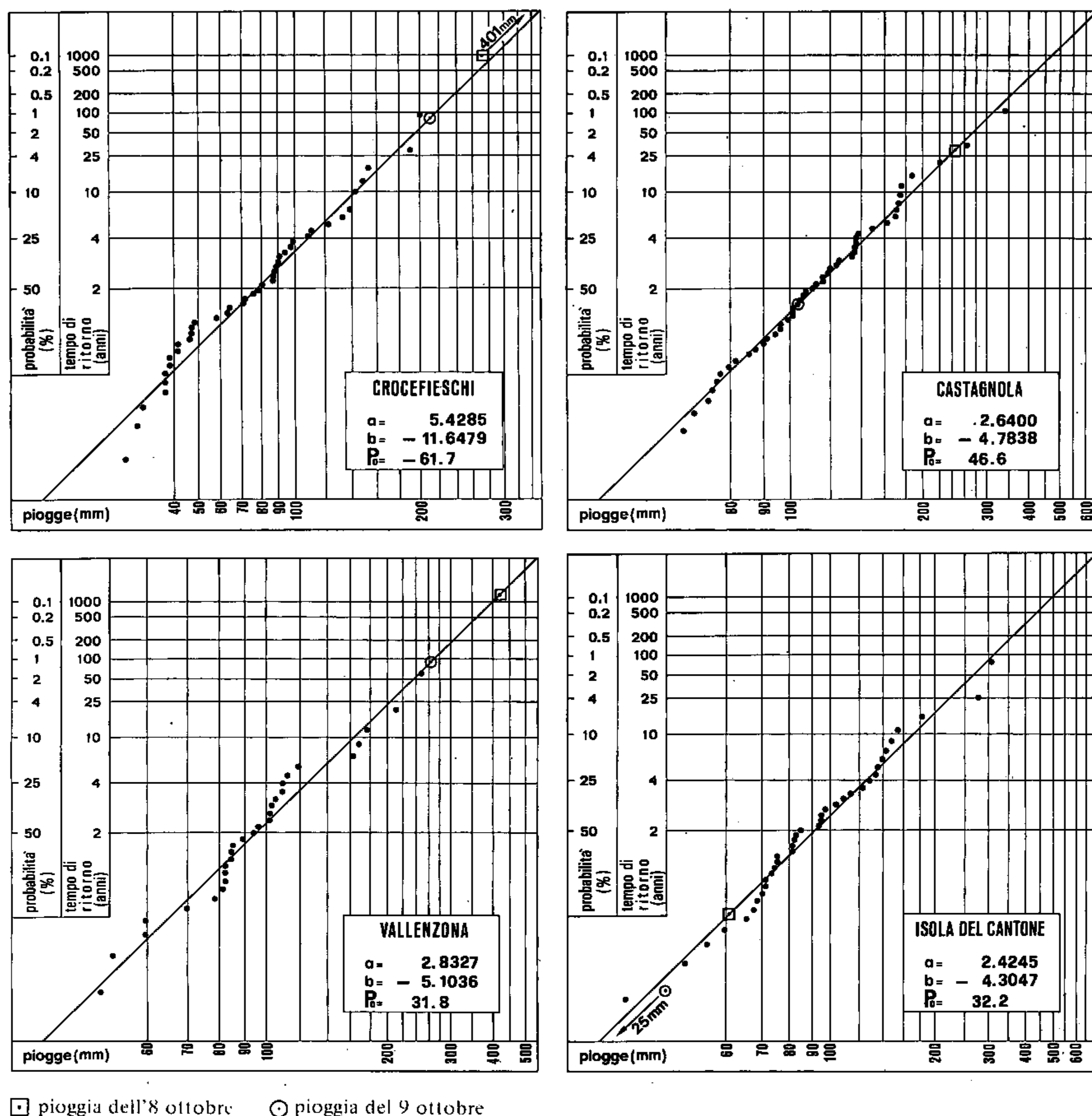
Fig. 5 - Regularizzazione secondo Gibrat delle piogge giornaliere delle stazioni di Crocefieschi, Castagnola, Vallenzone, Isola del Cantone.
