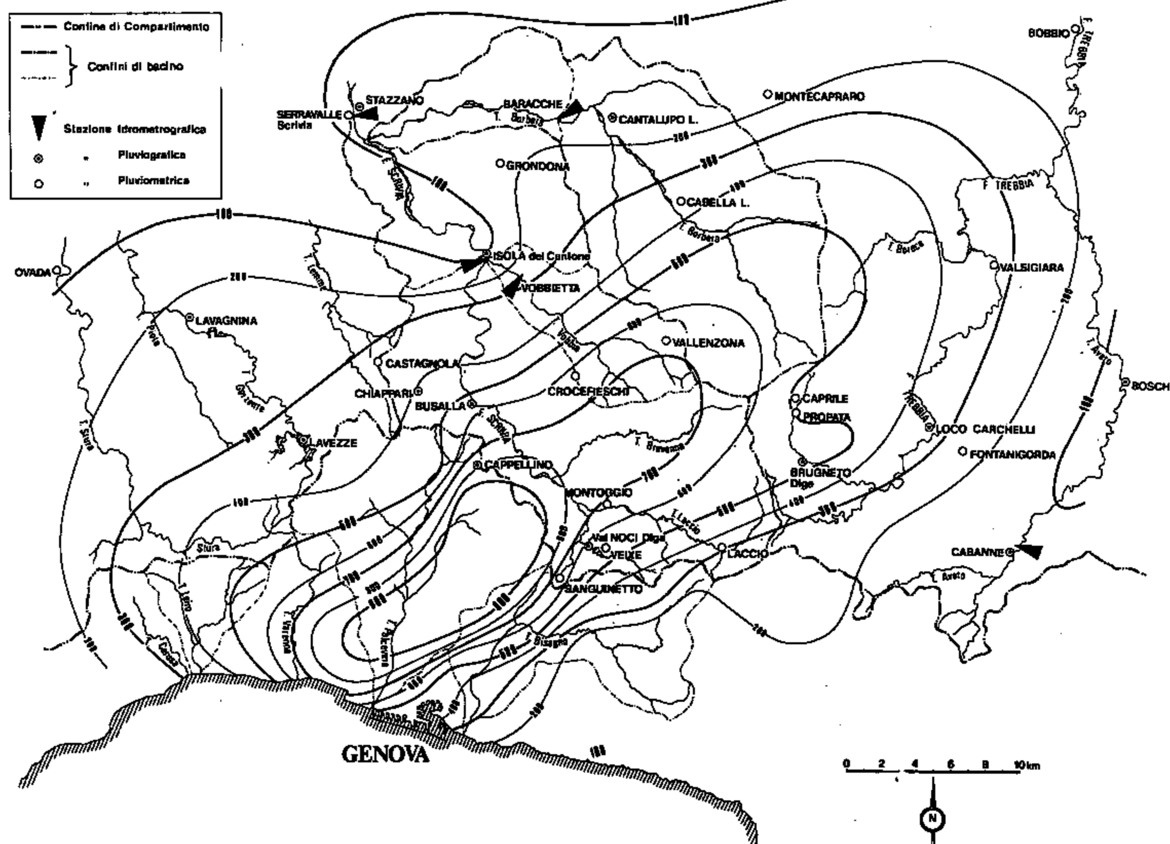
- Carta delle isoiete dei giorni 8 e 9 ottobre 1970
